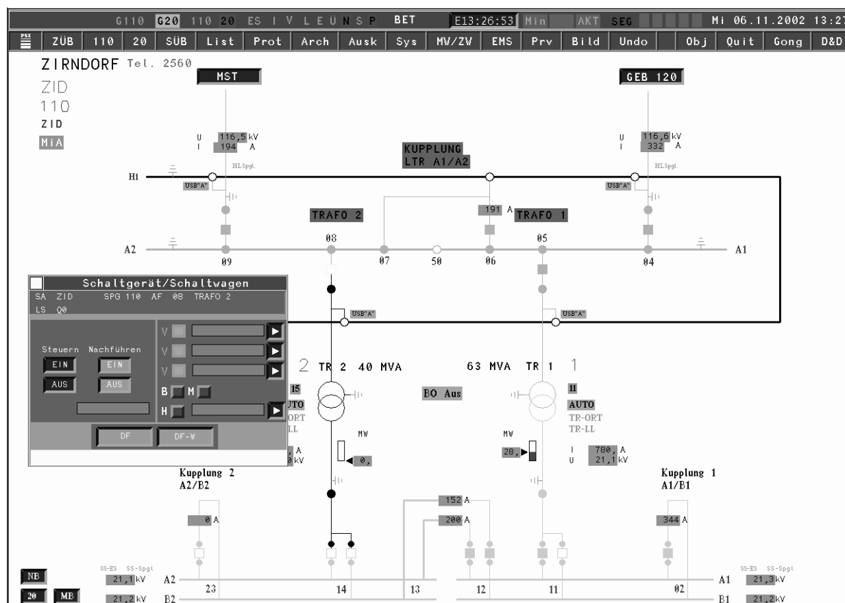
Abbildung 4.3: 110-kV-Anlagenbild
