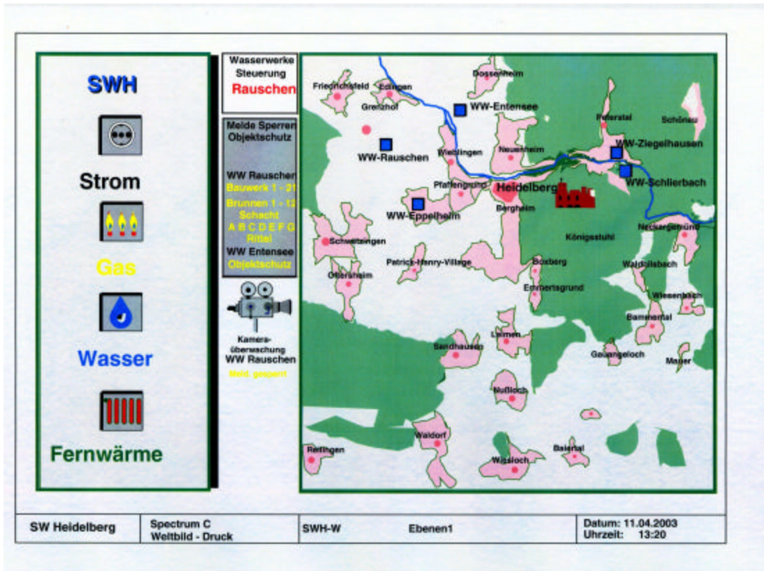
Abbildung A4.1: Übersichtsbild eines Querverbundleitsystems
