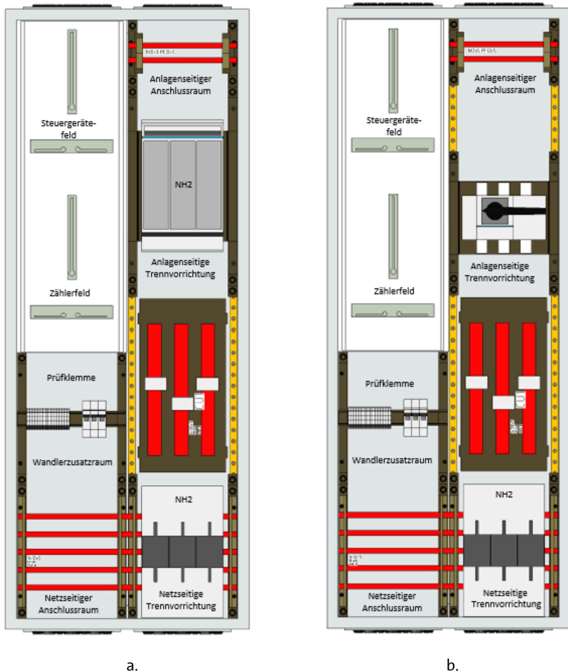
Abbildung 4: Beispiel für den Aufbau und Anordnung der Funktionsflächen einer Wandleranlage (Innenbe-reich, Standard-Kombischrank mit Höhe 1350mm) bei Bemessungsbetriebsströmen bis 200A nach DIN VDE 0603-2-2 im Versorgungsgebiet der ewk
