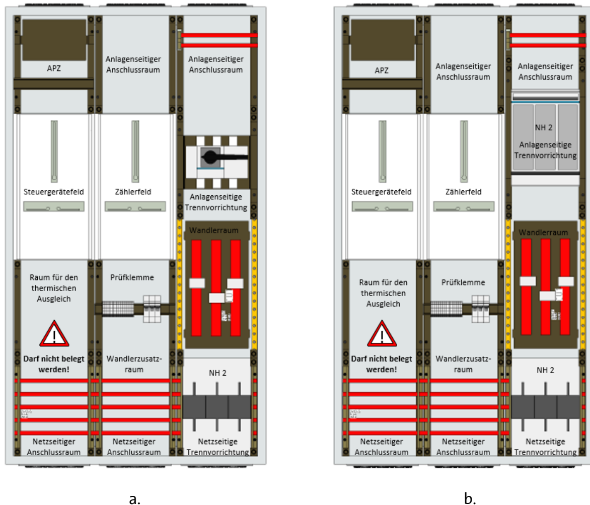
Abbildung 5: Beispiel für den Aufbau und Anordnung der Funktionsflächen einer Wandleranlage (Innenbe-reich, Standard-Kombischrank mit Höhe 1350mm) bei Bemessungsbetriebsströmen bis 250A nach DIN VDE 0603-2-2 im Versorgungsgebiet der ewk
